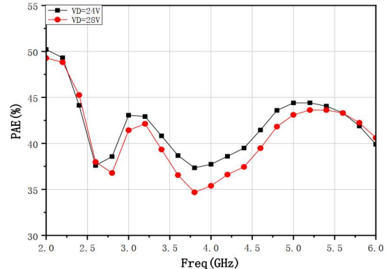
PAE
