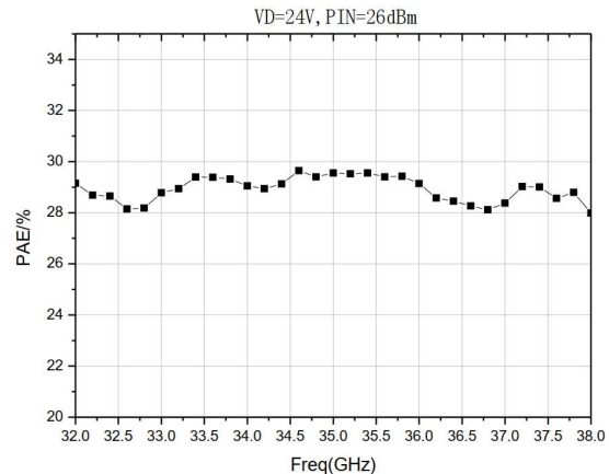
PAE
