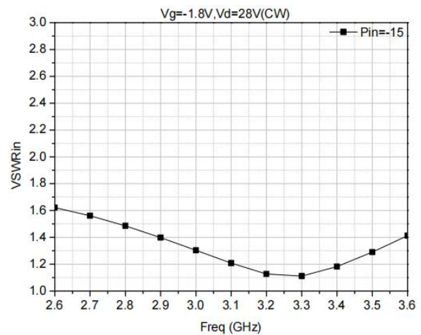
VSWRin
