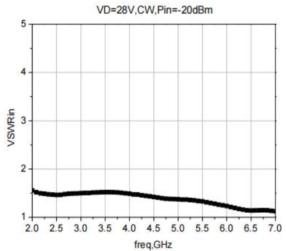
VSWRin
