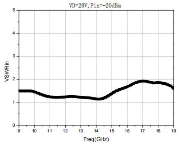
VSWRin
