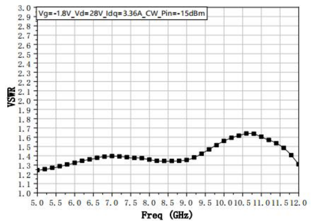
VSWRin
