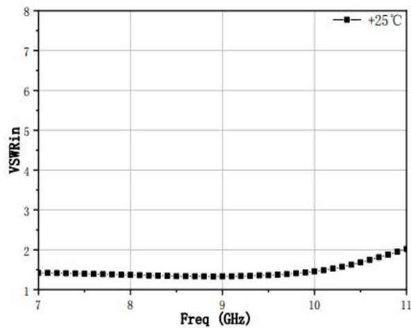
VSWRin
