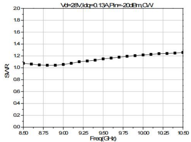
VSWRin
