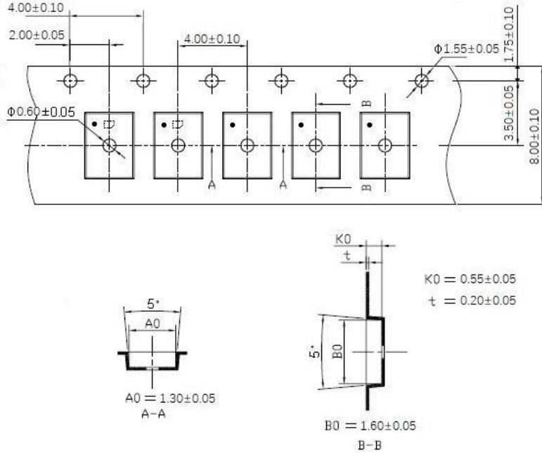
Reel Dimensions
