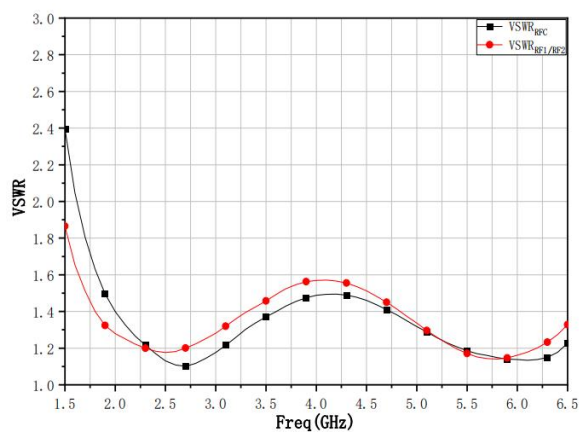
VSWR
