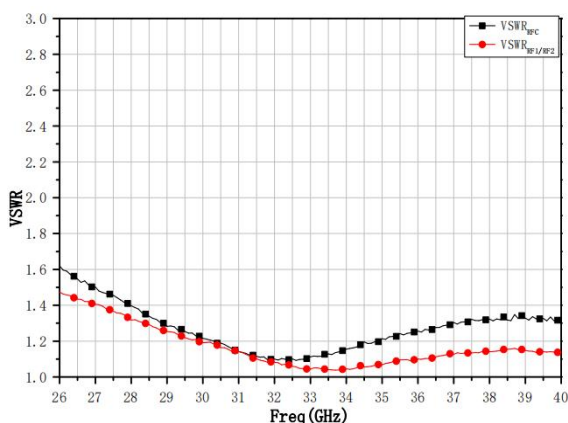
VSWR
