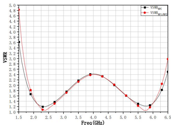
VSWR
