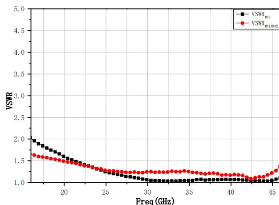
VSWR
