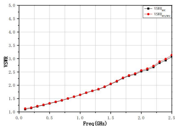
VSWR
