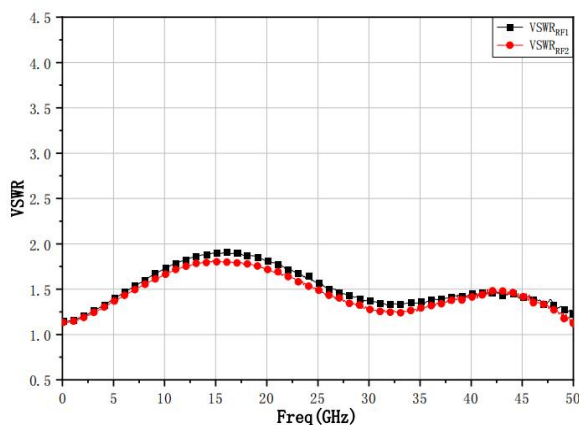
VSWR
