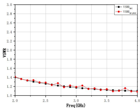
VSWR
