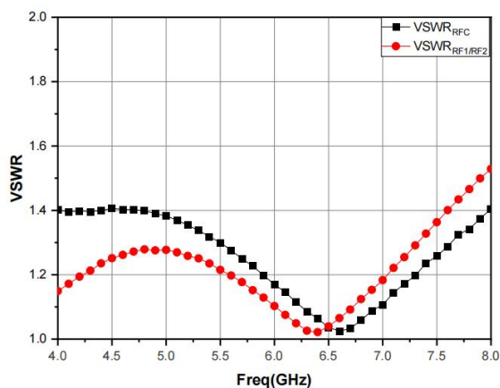
VSWR
