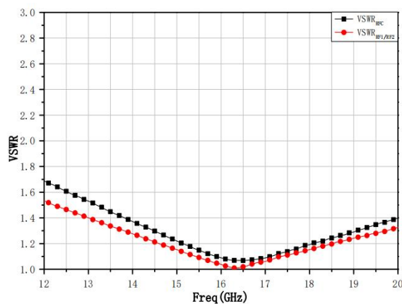
VSWR
