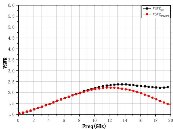
VSWR
