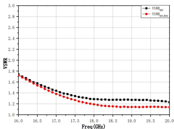
VSWR
