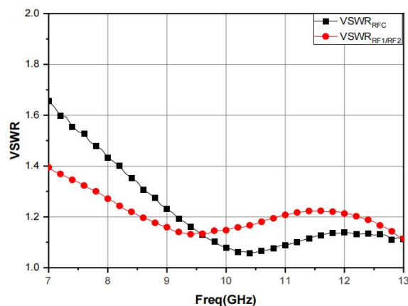
VSWR
