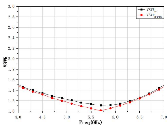
VSWR
