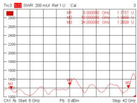
Output VSWR
