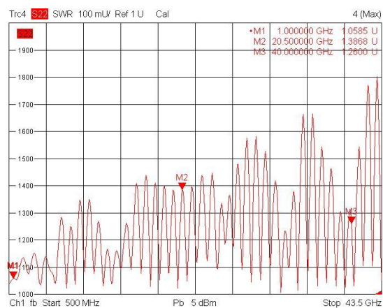
Output VSWR
