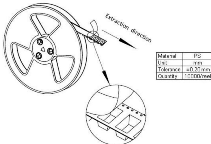
Reel Dimensions
