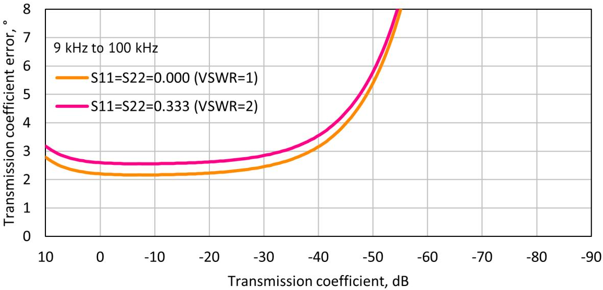
非匹配器件传输相位误差
